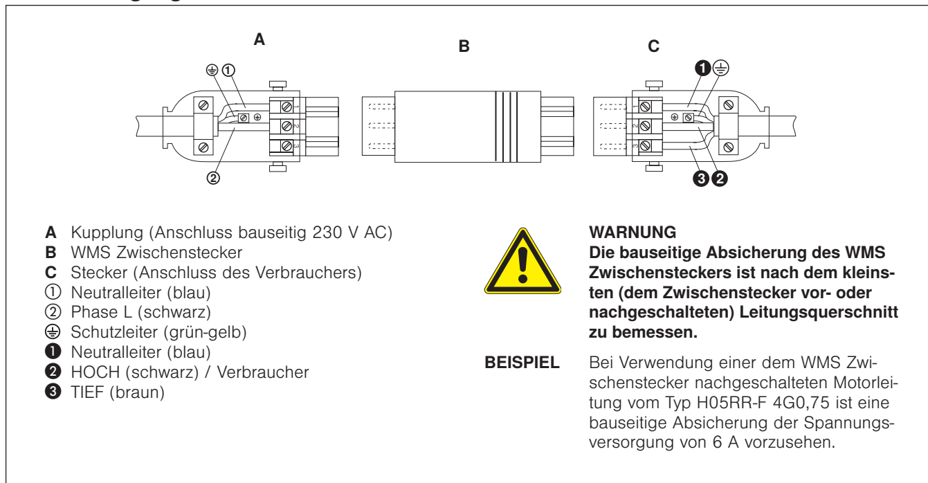
Abb. 2 Anschluss des Steckverbinders
