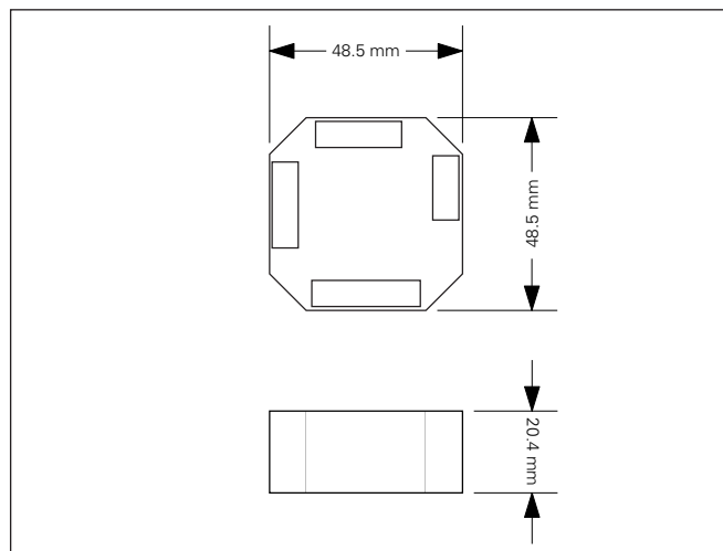
Abb. 3 Abmessungen
