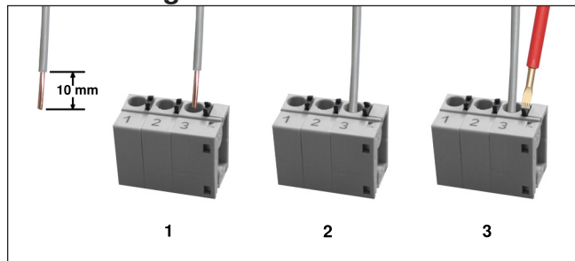
Abb. 2 Anschließen und Lösen der Leitungsverbindungen
