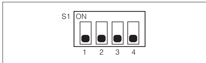
Abb. 2 Werkseinstellung Kodierschalter
