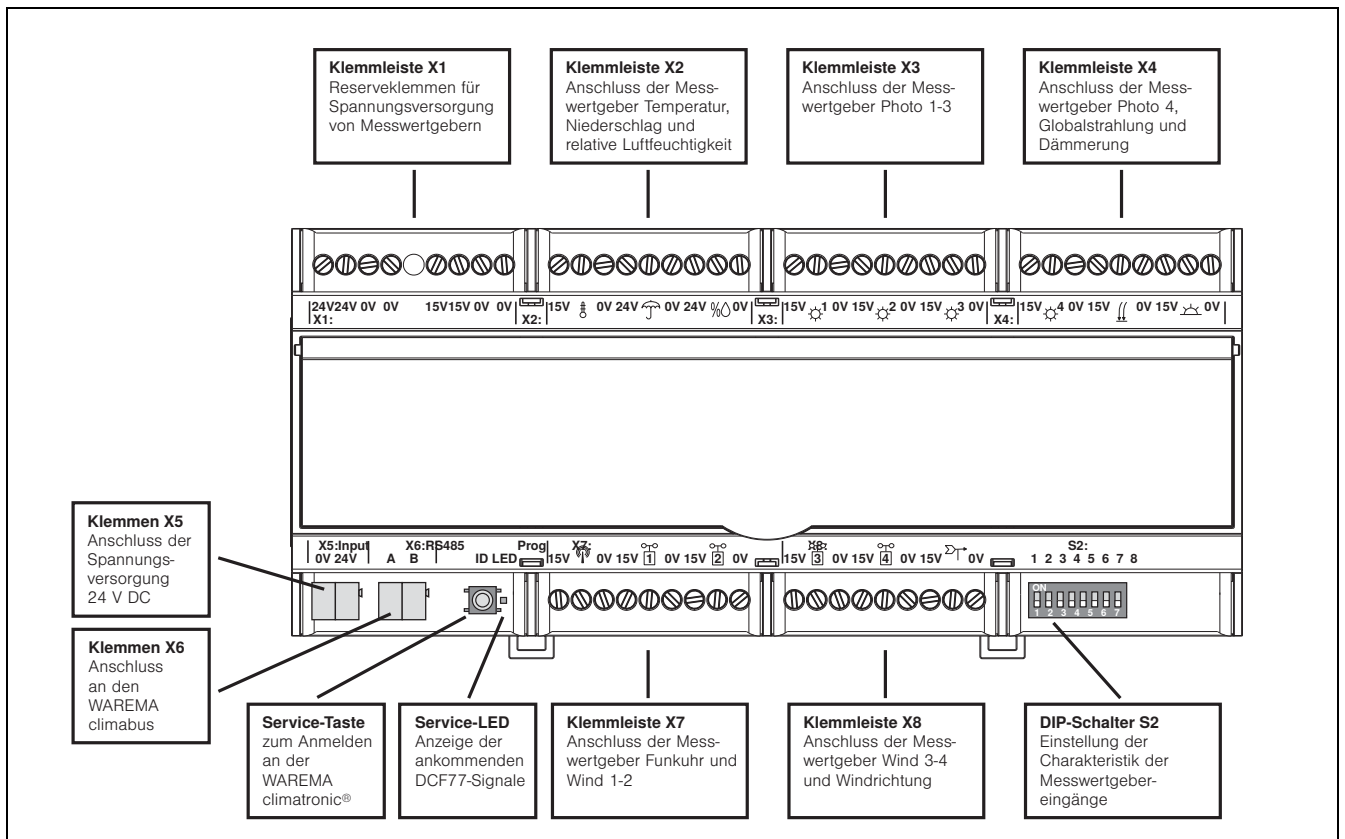
Abb. 120: Sensor Interface: Übersicht der Anschlussmöglichkeiten
