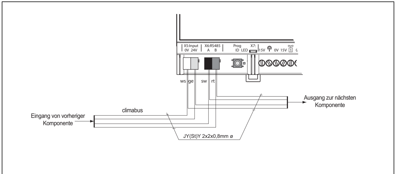
Abb. 119: Sensor Interface: Anschluss des climabus
